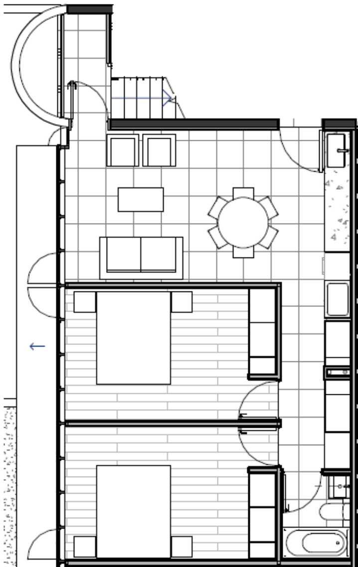
PLANO PISO 3
