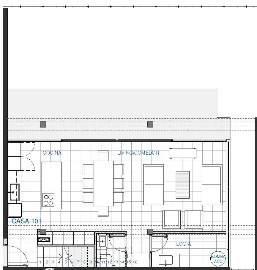
PLANO PISO 1
