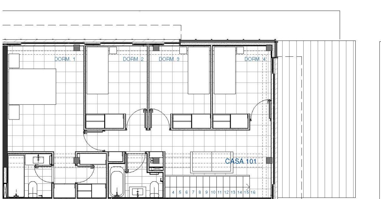
PLANO PISO 2
