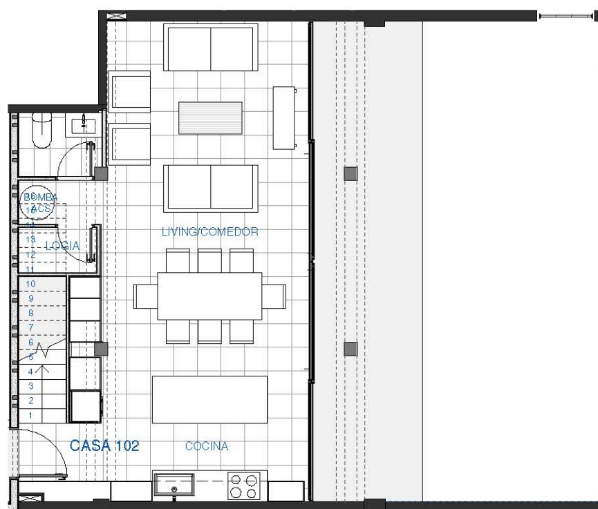
PLANO PISO 1
