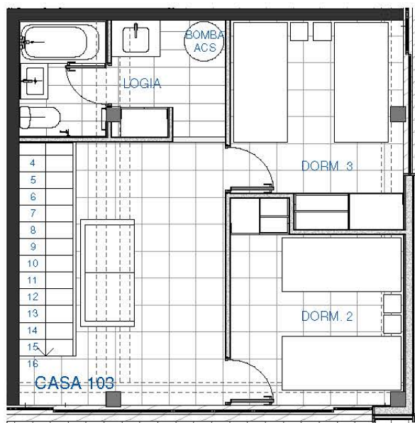
PLANO PISO 2
