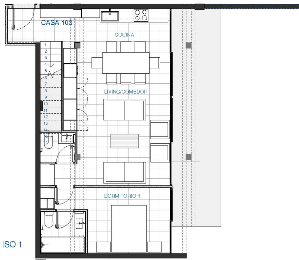
PLANO PISO 1
