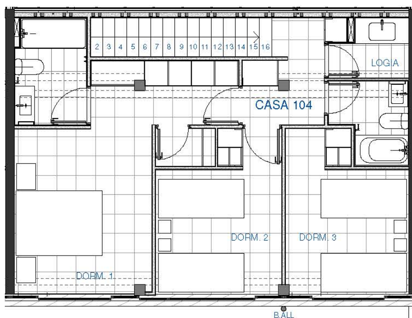
PLANO PISO 2
