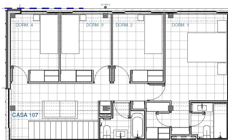
PLANO PISO 2
